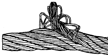
Рис. 11. Выдавливание сердечника
